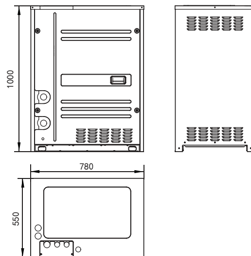
Figura 1. Tamanho da unidade externa
