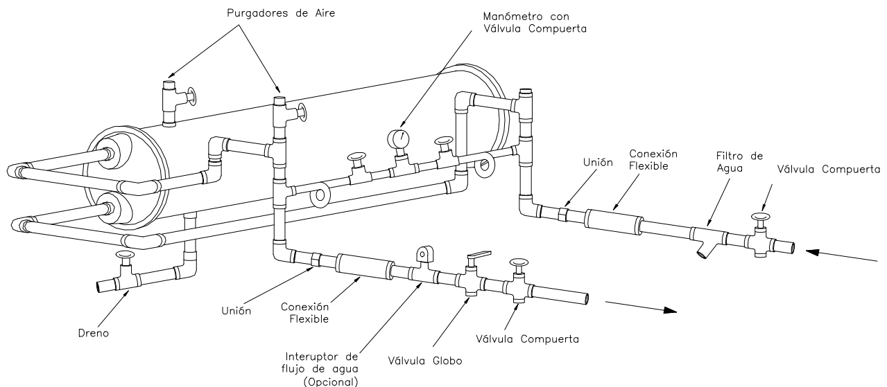
Fig. 5 - Componentes de la tubería hidráulica del evaporador
