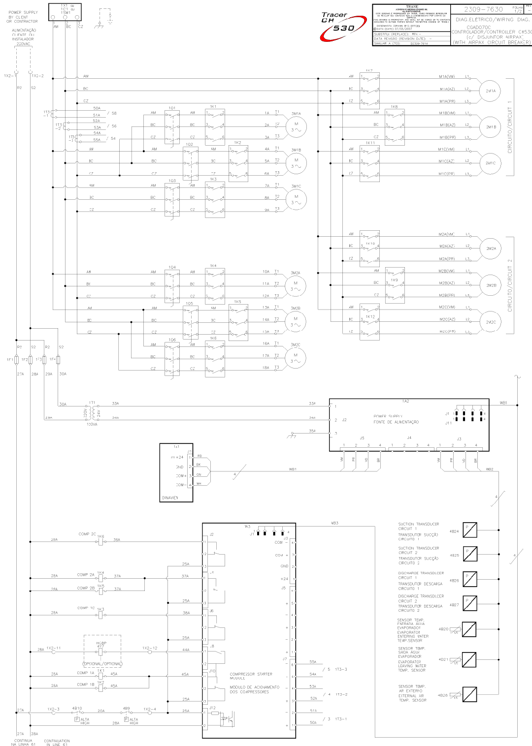
Fig. 26 - Diagrama Eléctrico - Fuerza y Comando CGAD 070C folha 1/2
