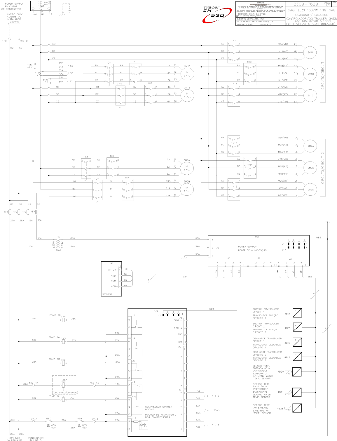
Fig. 23 - Diagrama Eléctrico - Fuerza y Comando CGAD 050C/060C folha 1/2
