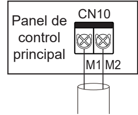
Conexión a unidad exterior M1M2 (HyperLink)
