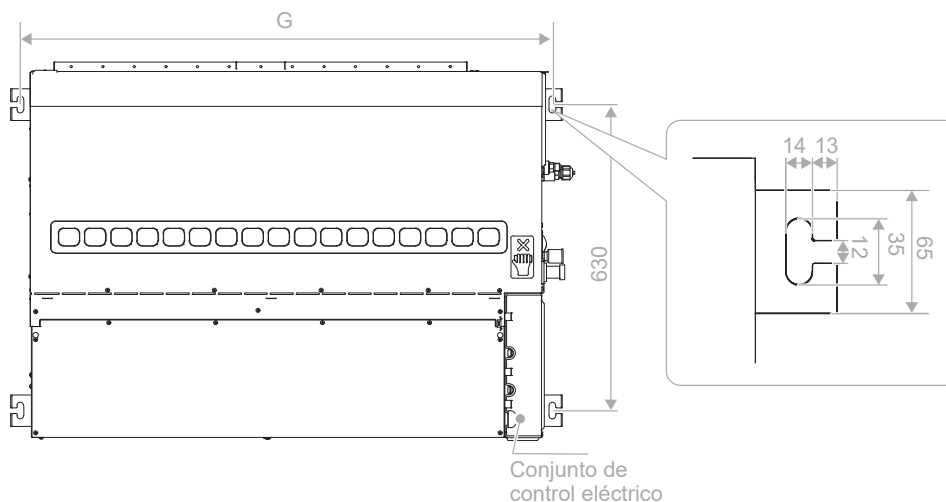
Tamaño de la entrada de aire de retorno y la distancia entre las terminales:
