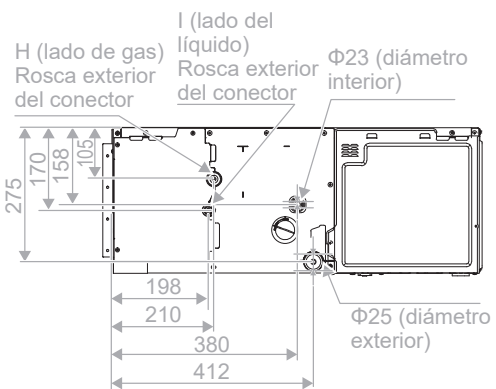
Dimensión de la tubería y tubería de agua:
