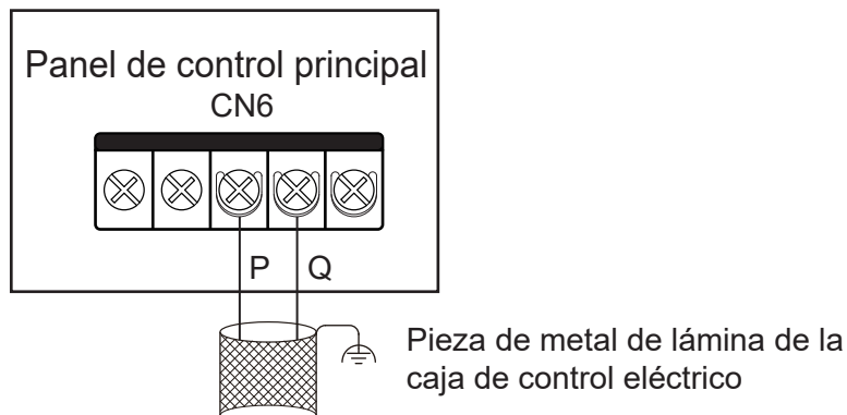
Conexión a la unidad exterior PQ
