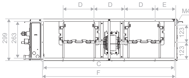
Tamaño de la entrada de aire de retorno y la distancia entre las terminales:
