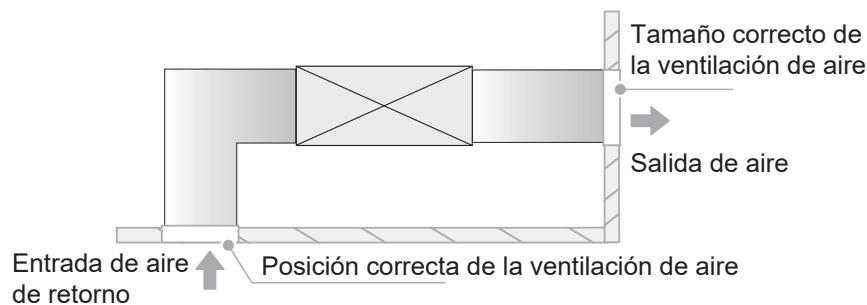
Tamaño y posición correctos de la ventilación de aire
