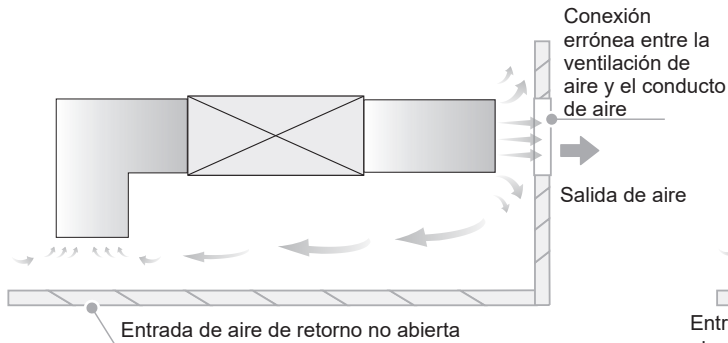
Conexión errónea entre la ventilación de aire y el conducto de aire
