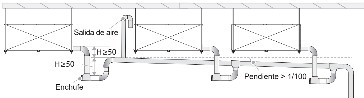
Método para conectar la tubería de drenaje para una unidad simple
