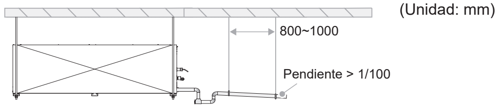
Método para conectar la tubería de drenaje para una unidad simple
