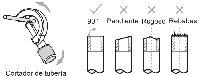
Cortador de tubería
