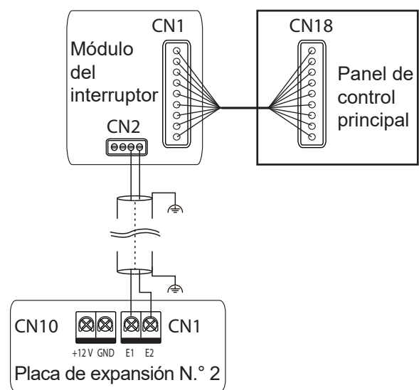
Use la placa de expansión N.º 2
