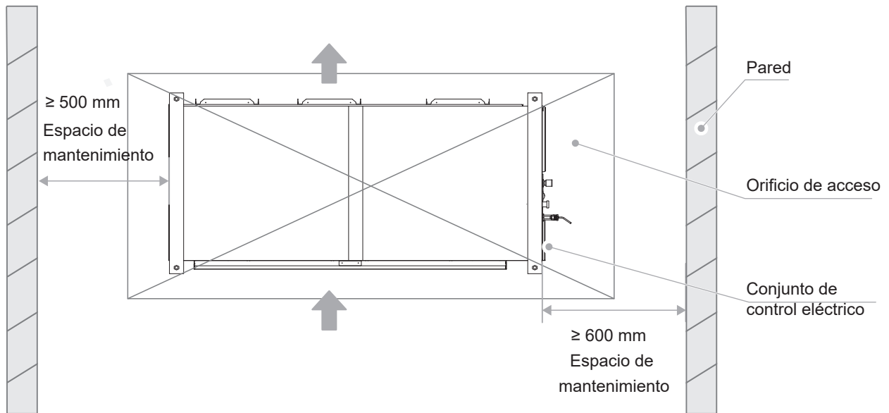
Vista inferior
